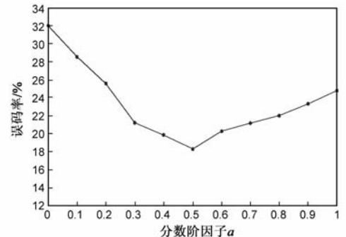
图5 白噪声环境下(10dB)不同分数阶因子 a 时的 3DFCCT 方法误码率曲线
