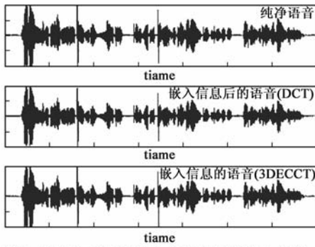
图2 离散余弦变换域上的低比特位嵌入方法
