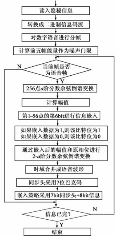
图1 离散分数余弦倒谱变换域上的低比特嵌入方法
